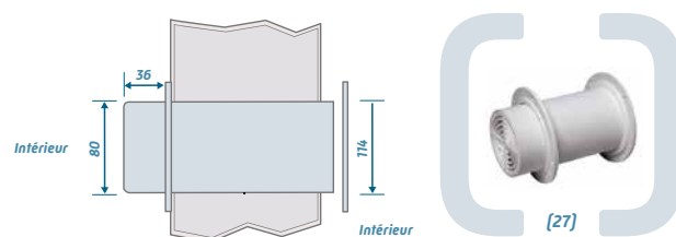
[27] Vanne d'équilibrage de pression T2-21
