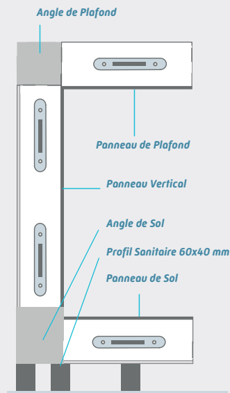
MATRIX 60, 85 et 105 - AVEC PLANCHER
