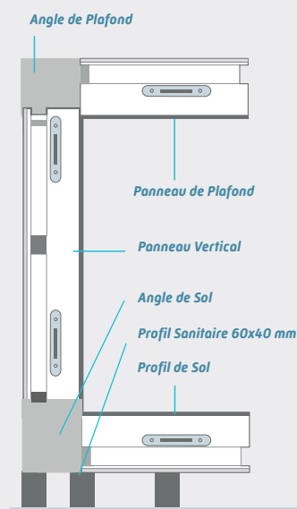
MATRIX 150 - AVEC PLANCHER
