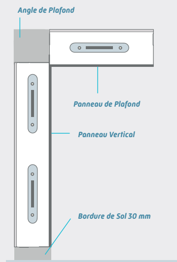
MATRIX 60, 85 et 105 - SANS PLANCHER
