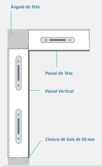
MATRIX 60, 85 e 105 - SEM SOLO
