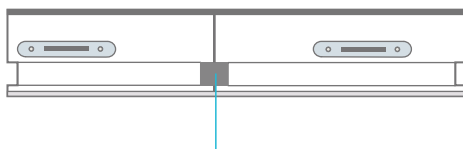
MATRIX 150: Isolamento de 30x20 mm entre 2 painéis
