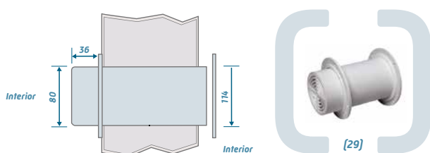
[29] Válvula de Equilíbrio de Pressão T2-21
