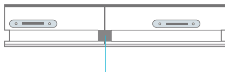
MATRIX 150: Aislamiento de 30x20 mm entre 2 paneles
