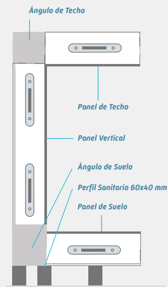
MATRIX 60, 85 y 105 - CON SUELO
