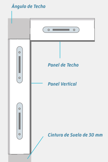
MATRIX 60, 85 y 105 - SIN SUELO
