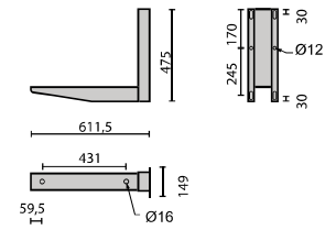
Suportes de parede - AAHS(PAR) - 80 L Wall brackets - AAHS(PAR) - 80L Système d'accrochage AAHS(PAR) - 80L
