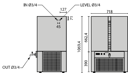
Arrefecedor de água - capacidade 120L Bakery water coolers - capacity 120L Refroidisseur d'eau - capacité 120L
