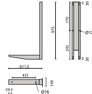
Suportes de parede - AAS(PAR) - 120L e 200L Wall brackets AAS(PAR) - 120L and 200L Système d'accrochage AAS(PAR) - 120L et 200L
