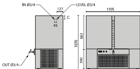
Arrefecedor de água - capacidade 200L Bakery water coolers - capacity 200L Refroidisseur d'eau - capacité 200L
