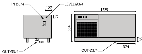
Arrefecedor de água - capacidade 80L Bakery water coolers - capacity 80L Refroidisseur d'eau - capacité 80L
