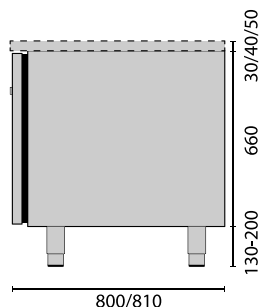
Porta aço inoxidável Doors in stainless steel Portes en inox
