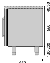
Porta de vidro Glass doors Portes en verre
