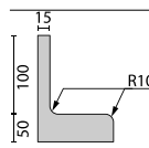
Tampo aço inoxidável c/ alçado Stainless steel top with splash-back Dessus acier inoxydable avec dossier
